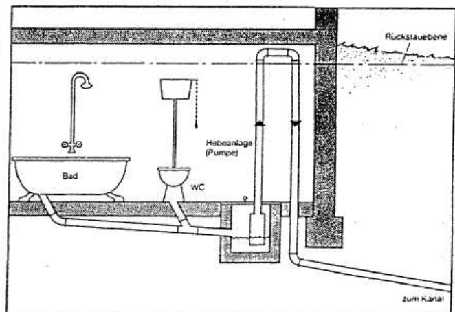
Bad und WC im Kellergeschoß mit Hebeanlage
