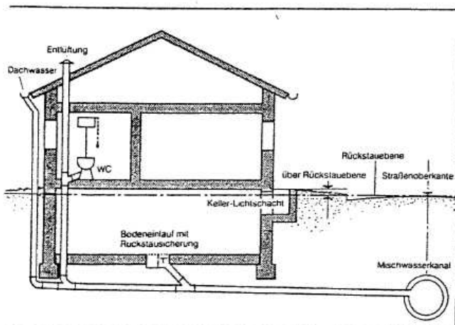
Sicherung des Kellergeschoßes gegen Überschwemmung
